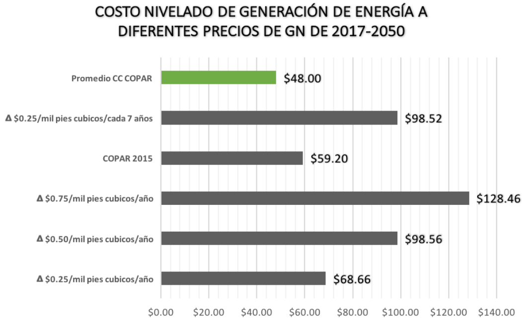
Figura 9. Costo nivelado de generación de energía a diferentes precios de gas natural de 2017 a 2050 ($USD/MWh)
